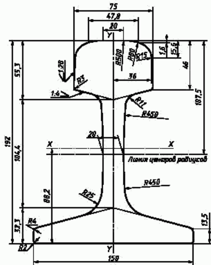
Рисунок А.4 — Рельс типа Р75
